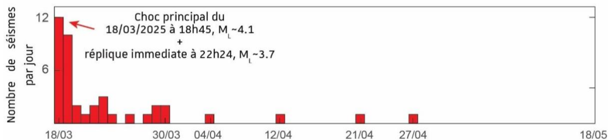
Figure 2-2 Sismicité dans un rayon de 5 km autour de l'épicentre du séisme du 18 mars 2025 enregistrée par le BCSF-Rénass entre juillet 2020 et juillet 2025. En rouge, la sismicité enregistrée du 18/03/2025 au 08/07/2025. La zone considérée affiche un faible taux de sismicité avant le choc principal, sans indications d'événements précurseurs. Près de 40 répliques ont été enregistrées durant le mois suivant cet événement. (B. Derodes, ITES 2025).
