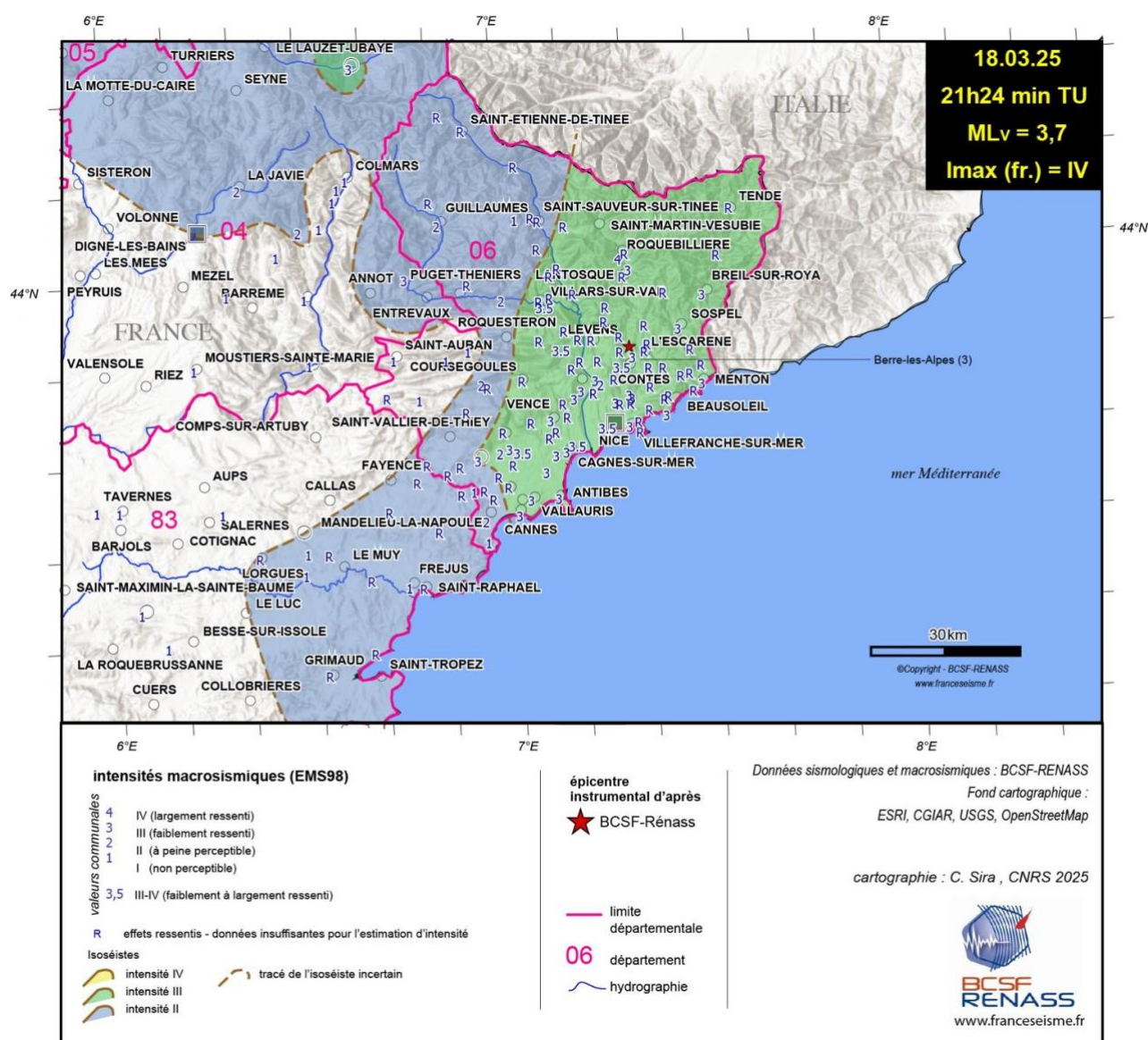
Figure 3-4 Carte d'intensités macrosismiques EMS-98 du séisme du 18 mars 2025 à 22h24 locale, réalisée d'après les formulaires communaux, complétées des informations individuelles reçues sur www.franceseisme.fr .
