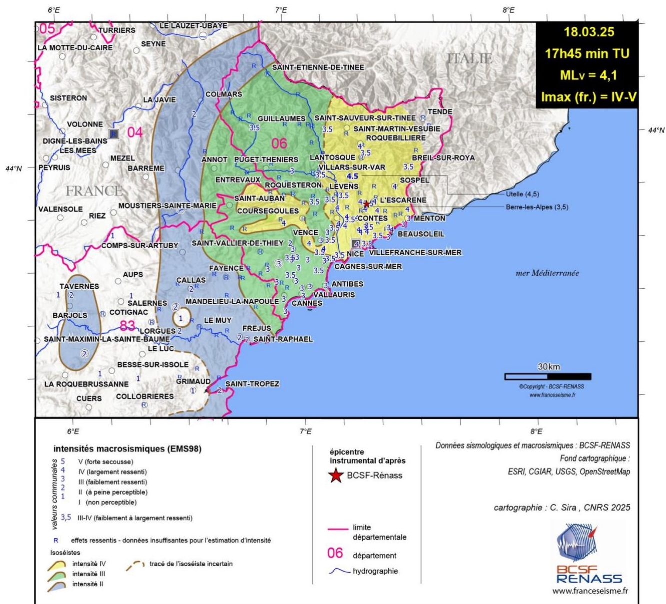
Figure 3-1 Carte d'intensités macrosismiques EMS-98 (18/03/2025 – 17h45 TU, 4,1 M_L ), réalisée d'après les formulaires communaux, complétée des informations individuelles reçues sur www.franceseisme.fr .
