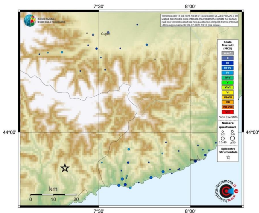
Figure 3-2 Carte d'intensités automatiques de l'INGV (répartition de l'intensité des secousses sismiques dans la région, exprimée en termes d'intensité sur l'échelle MCS (Mercalli-Cancani-Sieberg). Les intensités sont déterminées à partir des données issues des questionnaires recueillis sur le site web http://www.hsit.it , en tenant compte de tous les rapports reçus de chaque commune et sont d'autant plus fiables que le nombre de questionnaires est élevé. Les données collectées sont soumises à un filtre statistique automatique, mais ne sont pas vérifiées individuellement).
