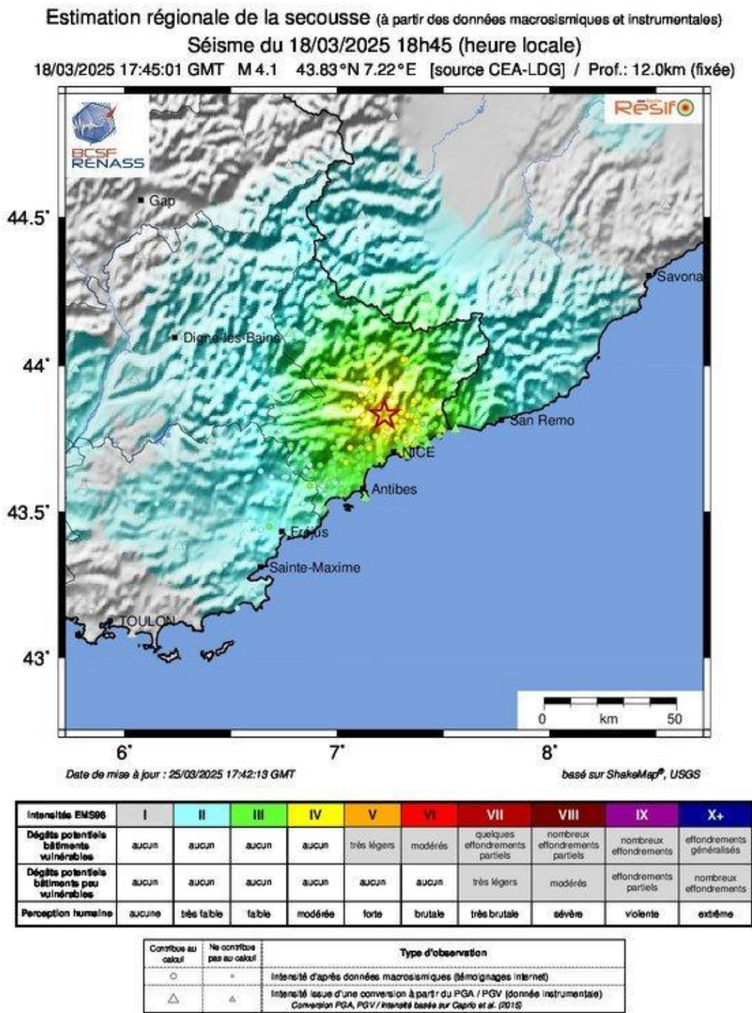
Cartes de modélisation de la secousse
