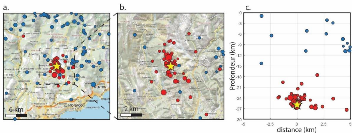
Figure 2-1 Sismicité autour de l'épicentre du séisme du 18 mars 2025 enregistrée par le BCSF-Rénass ces 5 dernières années (08/07/2020 – 08/07/2025). a. Carré de 30 km de côté centré sur l'événement principal. b. Carré de 10 km de côté centré sur l'événement principal. c. Vue en coupe Ouest-Est de la sismicité en b. En bleu clair les séismes du 08/07/2020 au 18/03/2025, en rouge les séismes depuis le choc principal, du 18/03/2025 au 08/07/2025 (B. Derodes, ITES 2025).
