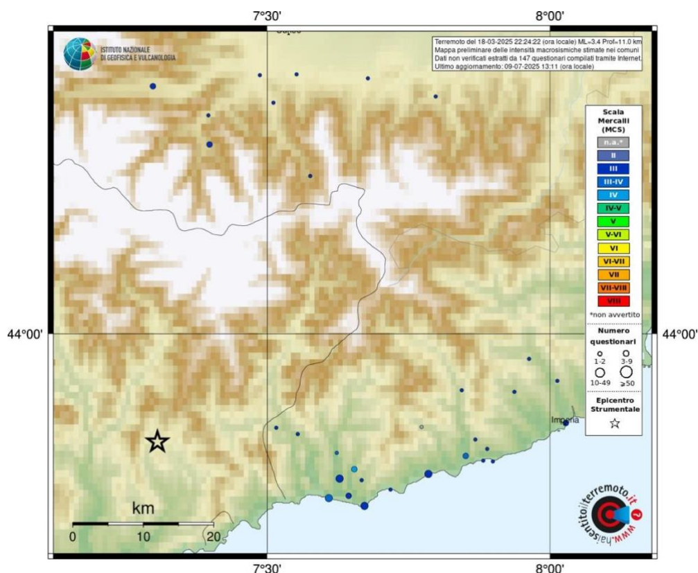
Figure 3-6 Carte d'intensités automatiques du séisme du 18 mars 2025 à 22h24 locale, réalisée par l'INGV (intensité des secousses sismiques exprimée en termes d'intensité sur l'échelle MCS (Mercalli-Cancani-Sieberg)). Les intensités sont déterminées à partir des données issues des questionnaires recueillis sur le site web http://www.hsit.it , en tenant compte de tous les rapports reçus de chaque commune et sont d'autant plus fiables que le nombre de questionnaires est élevé. Les données collectées sont soumises à un filtre statistique automatique, mais ne sont pas vérifiées individuellement).
