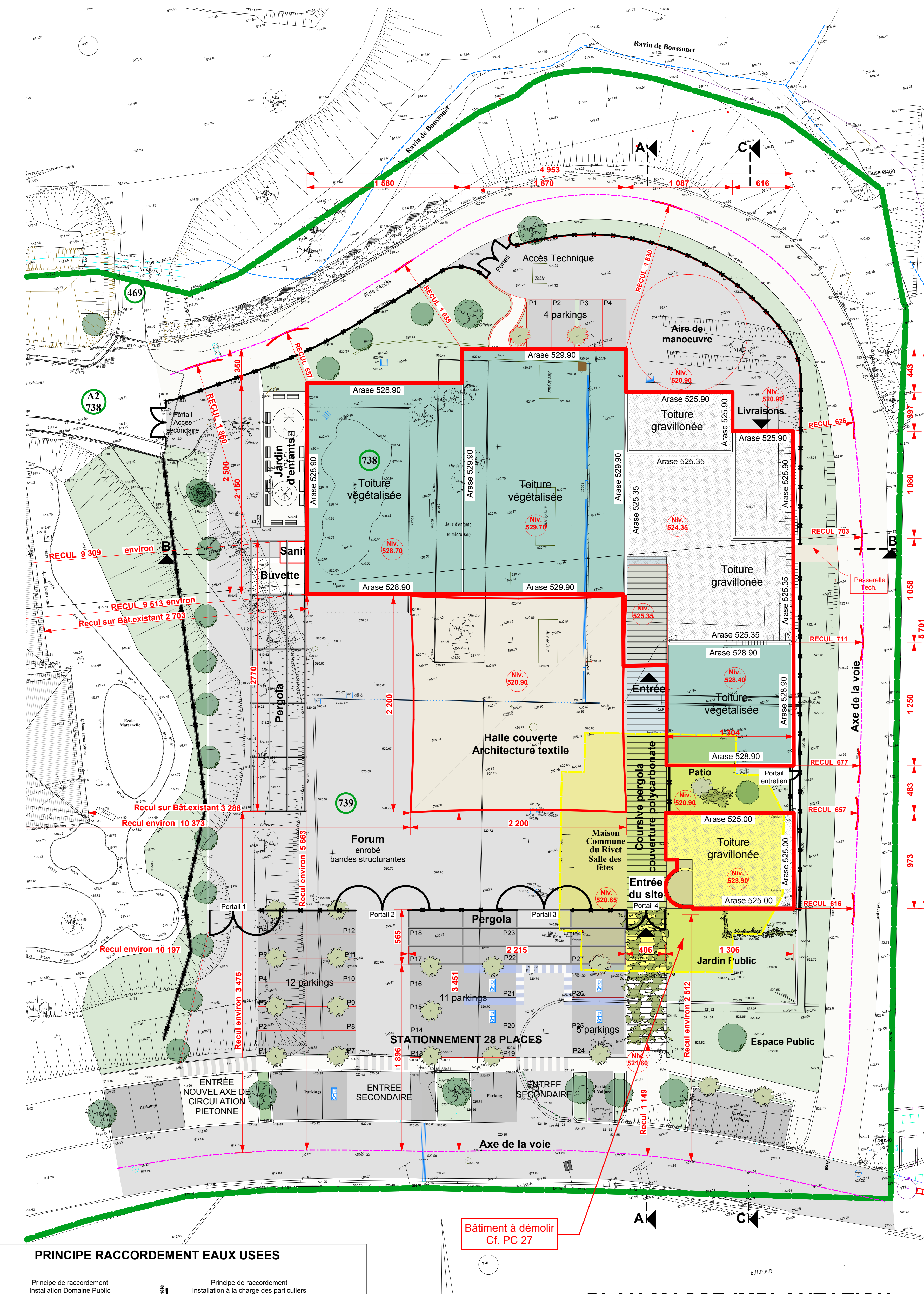
PLAN MASSE IMPLANTATION Ech: 1/200
