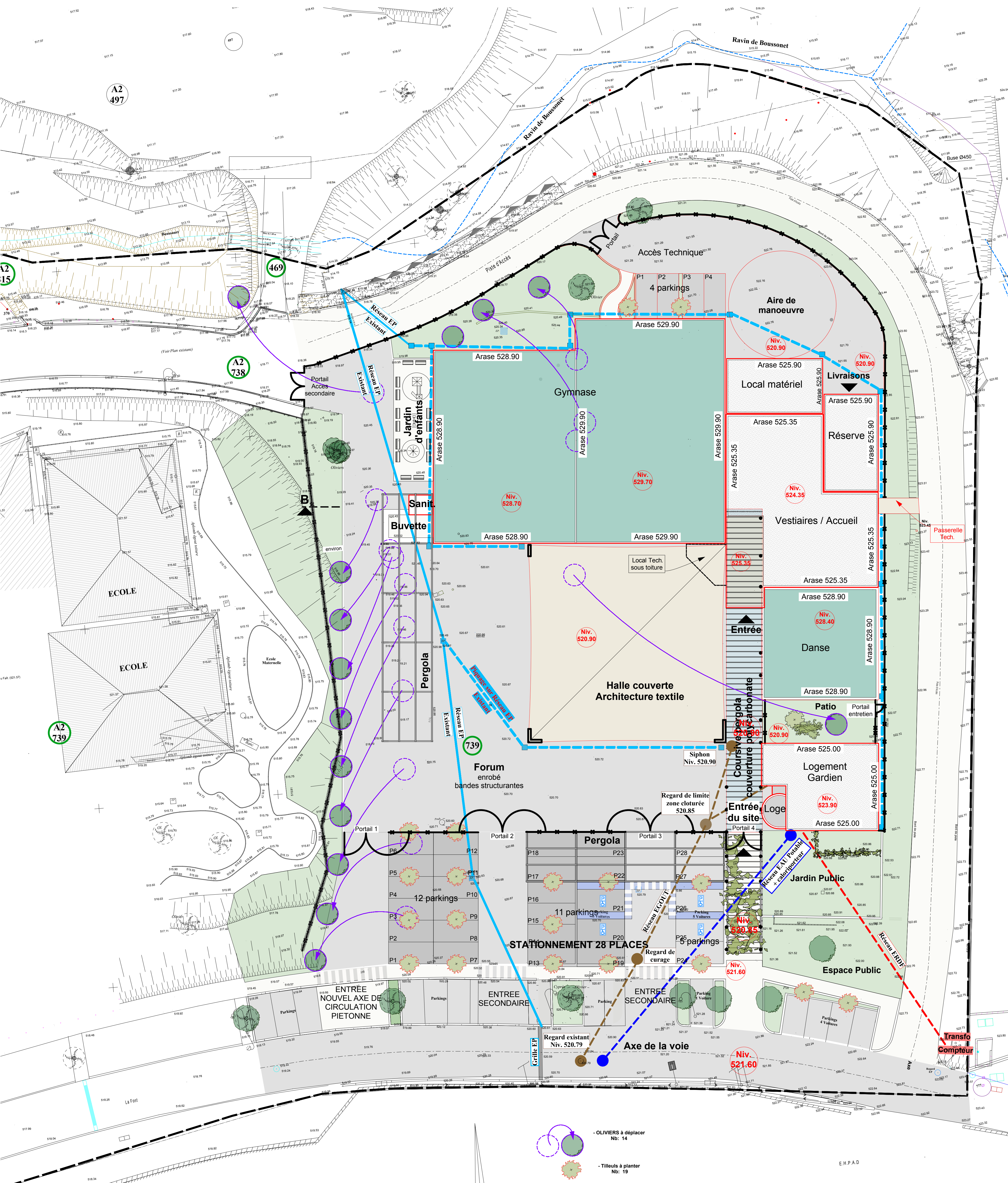
PLAN MASSE RESEAUX / PAYSAGE Ech: 1/200
