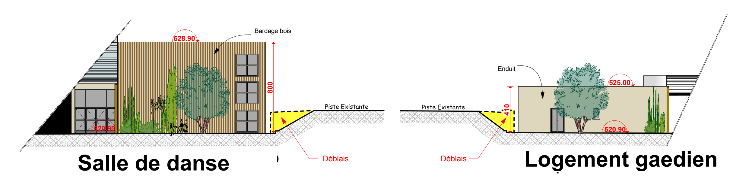
Façades depuis Patio Ech: 1/200
